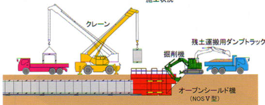
施工状況
