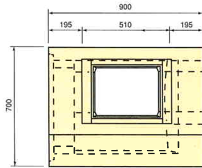
中央断面図
