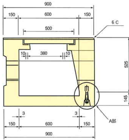
中央断面図
